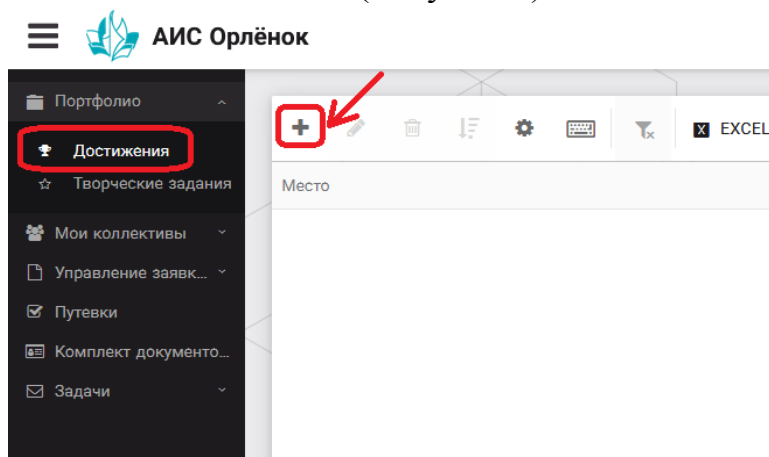
Рисунок 4 – Загрузка достижений
